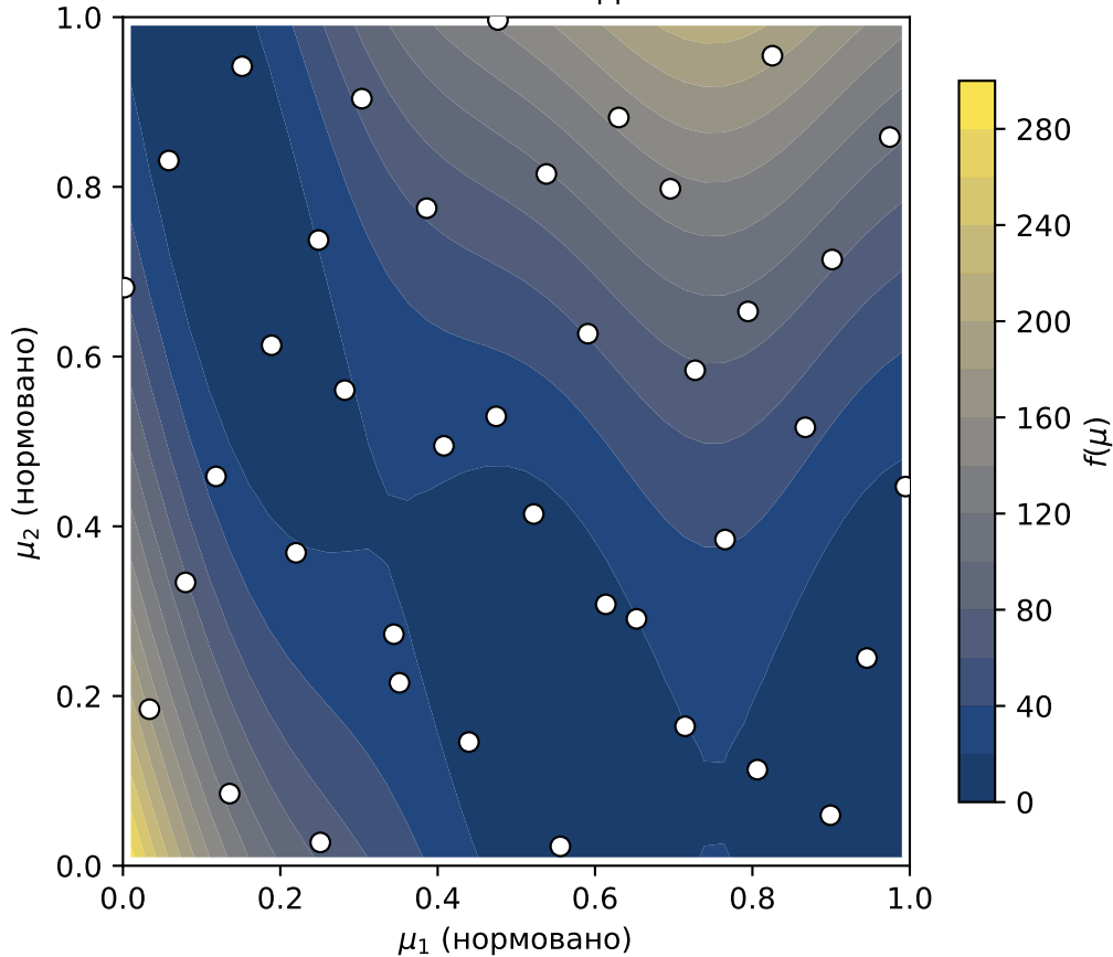
LHS: 40 точок на задачі branin
